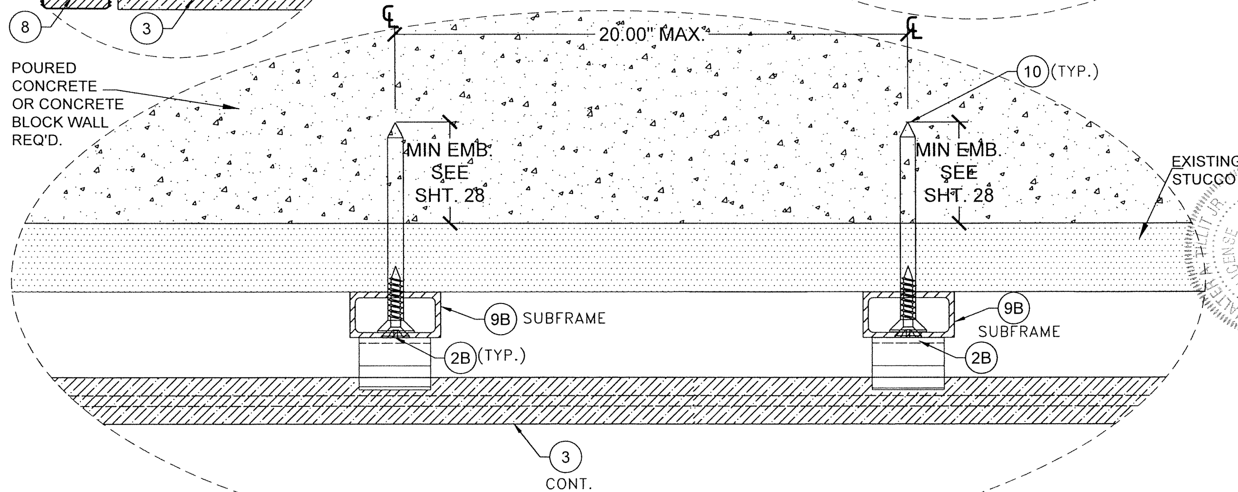
DETAIL 2 N.T.S.
