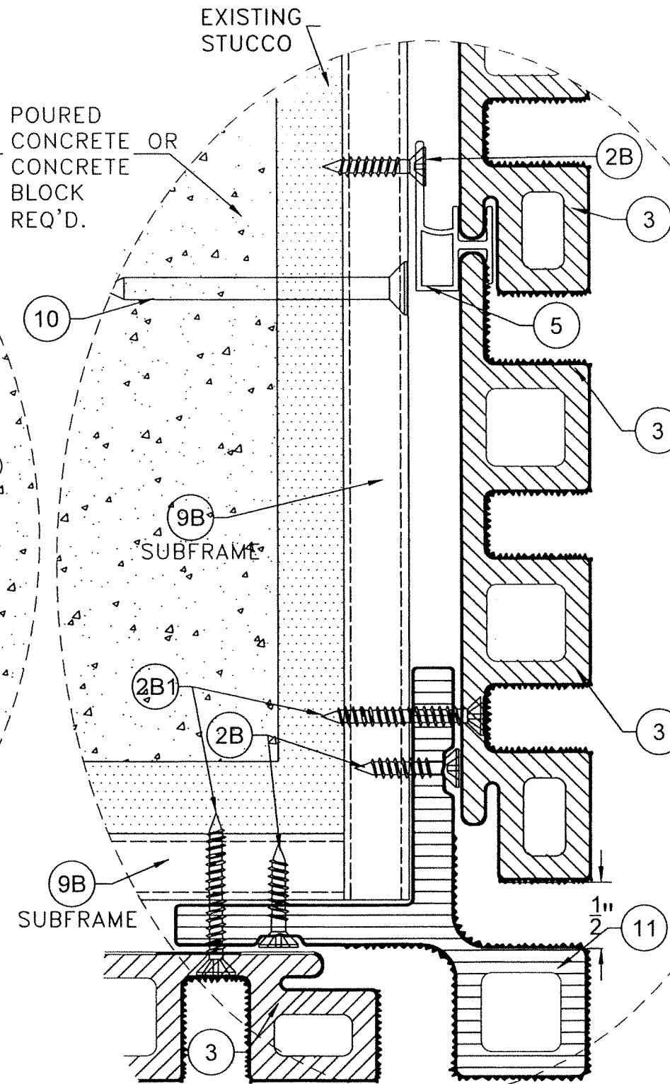
DETAIL 5 N.T.S.
