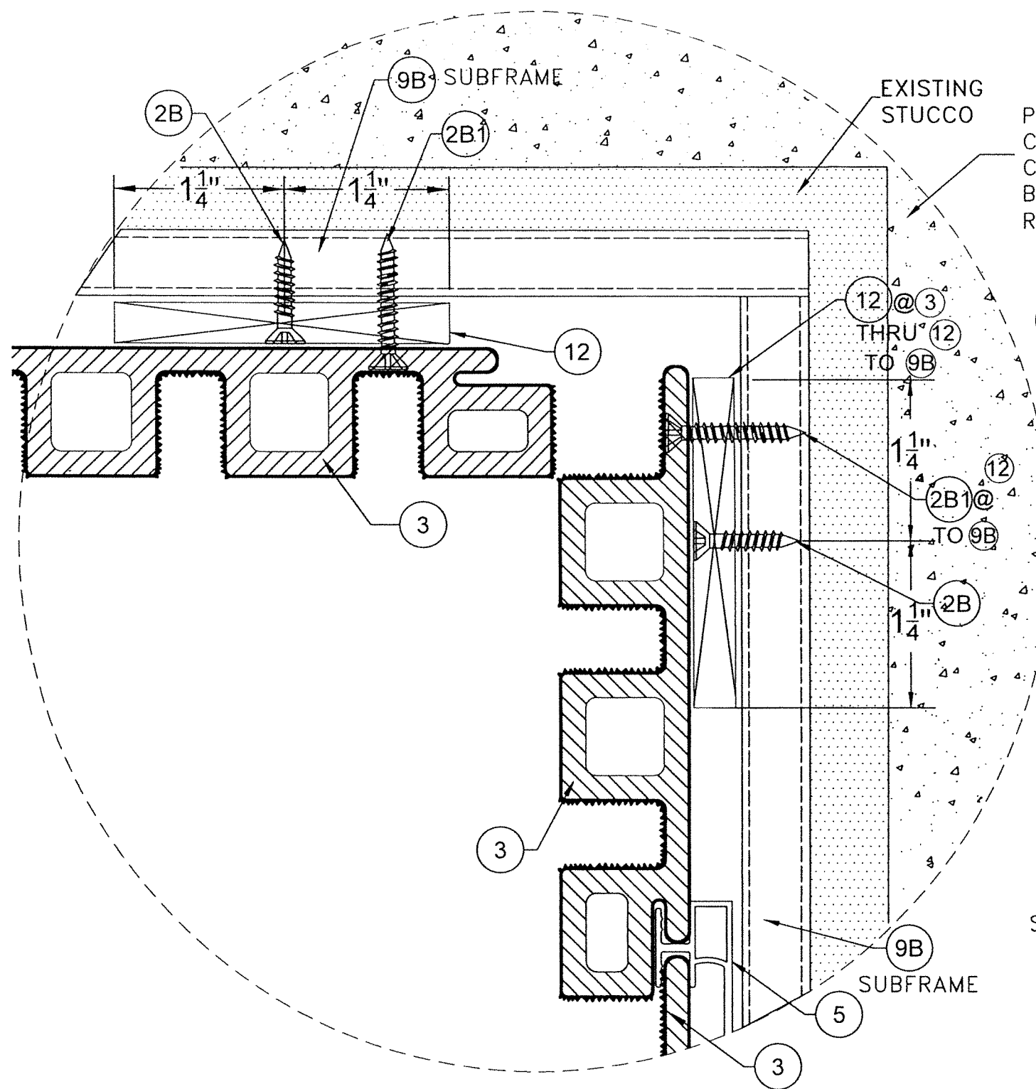
DETAIL 4 N.T.S.
